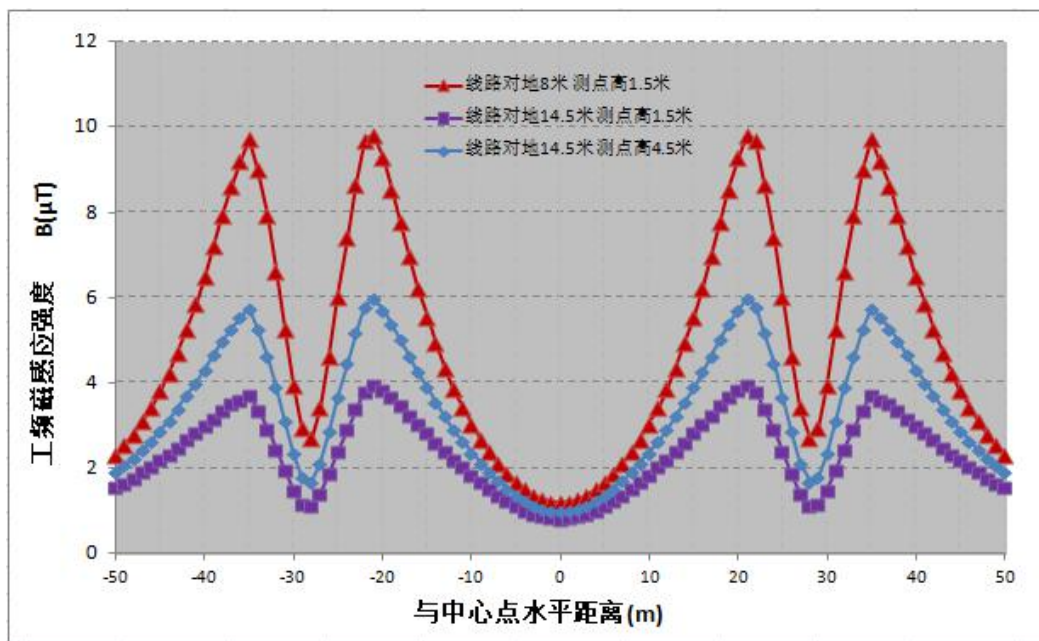
图 6.1-21 工频磁感应强度分布曲线图
