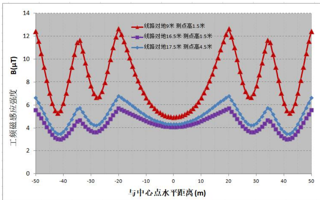
图 6.-15 工频磁感应强度分布曲线图
