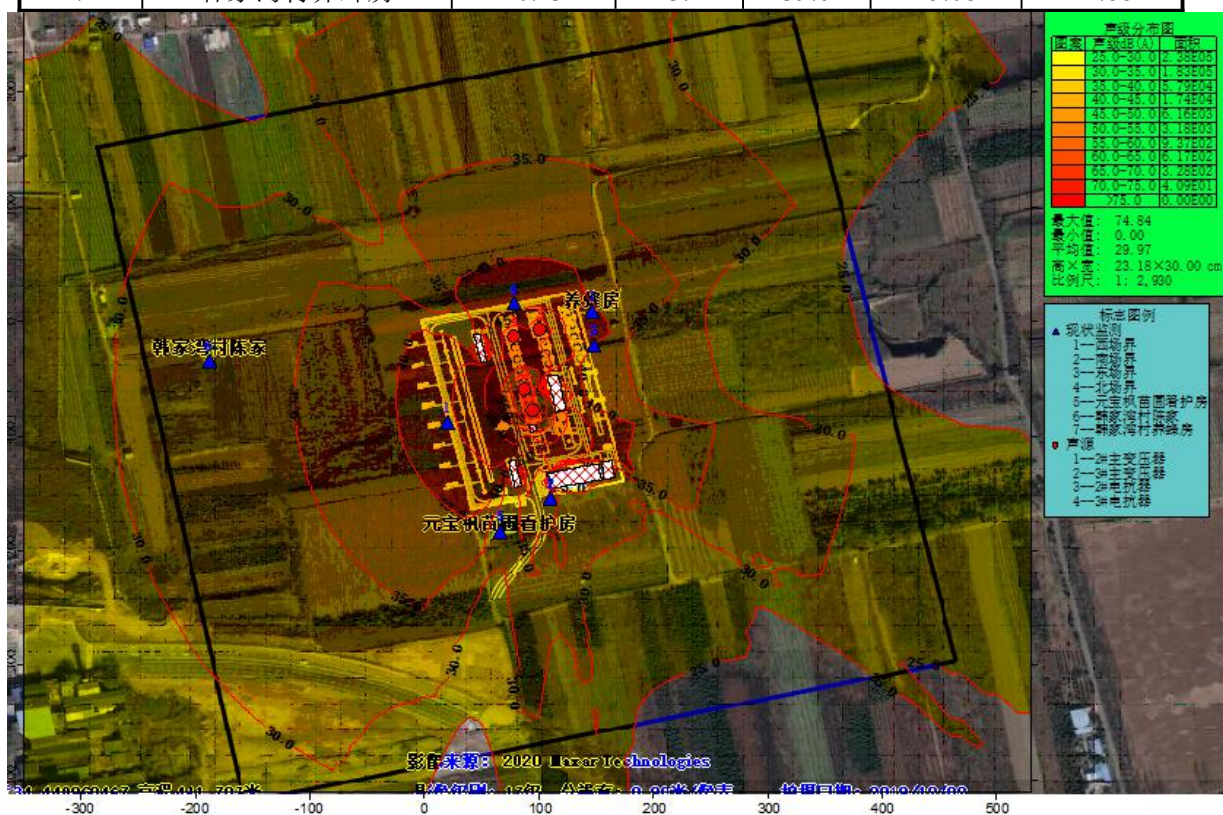
图 6.2-1 咸阳东 330kV 变电站等效噪声级预测
