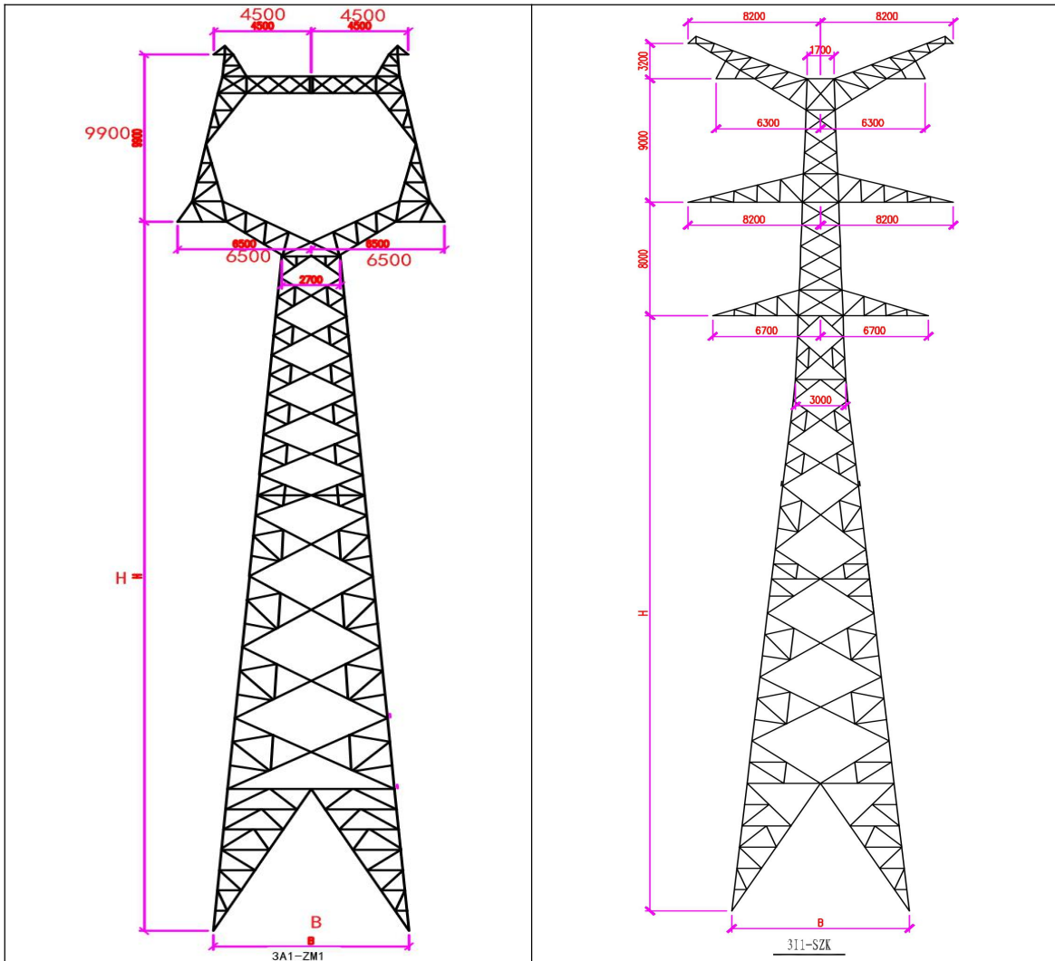
图 6.1-7 计算示意图
