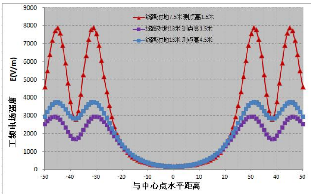
图 6.1-18 工频电场强度分布曲线图
