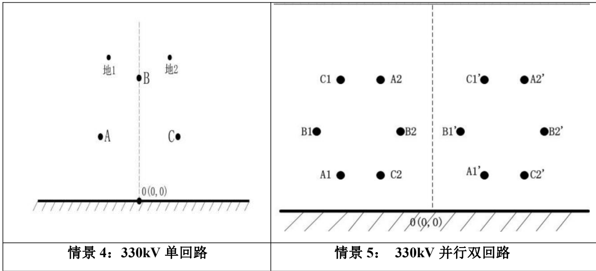
图 6.1-7 计算示意图
