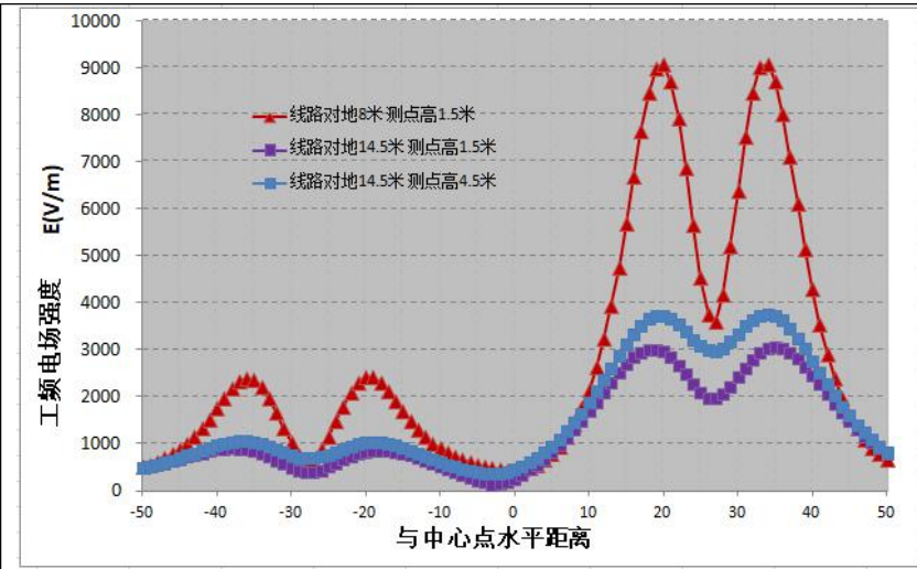
图 6.1-22 工频电场强度分布曲线图
