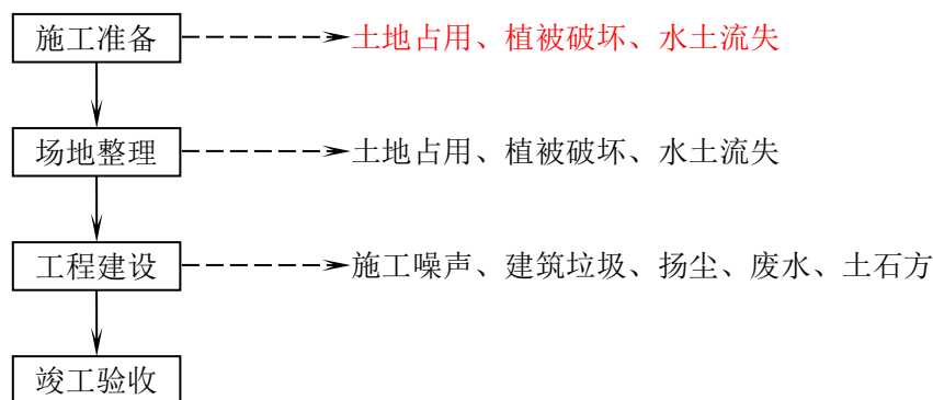
图 3.2-1 变电站建设施工工艺及产污环节
