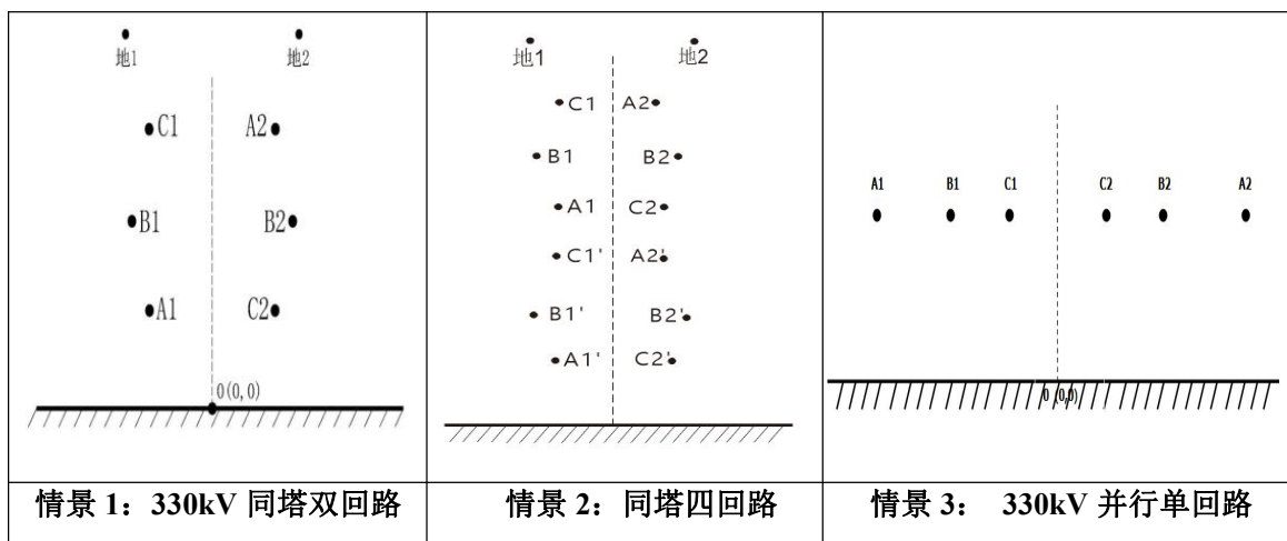
图 6.1-5 计算示意图
