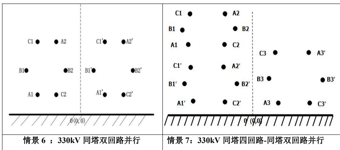
图 6.1-9 计算示意图
