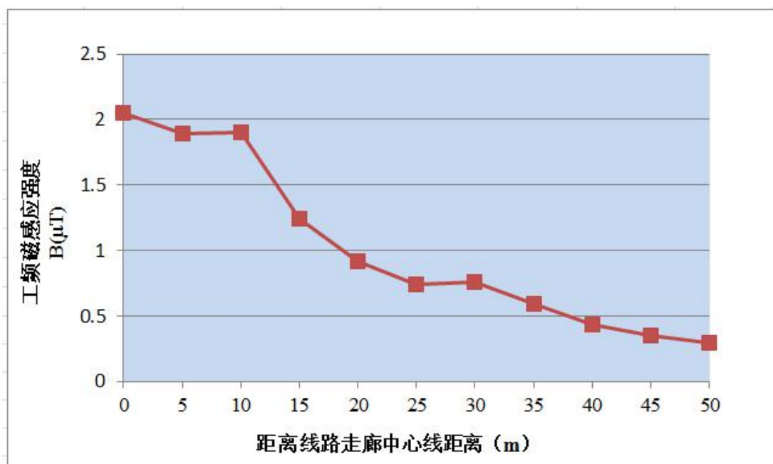
图 6.1-26 类比双回线路工频磁感应强度分布图
