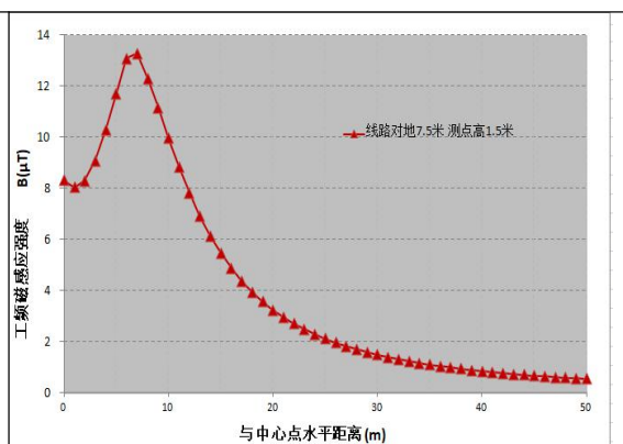
图 6.1-17 工频磁感应强度分布曲线图
