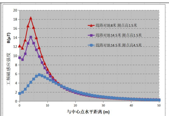
图 6.1-11 工频磁感应强度分布曲线图
