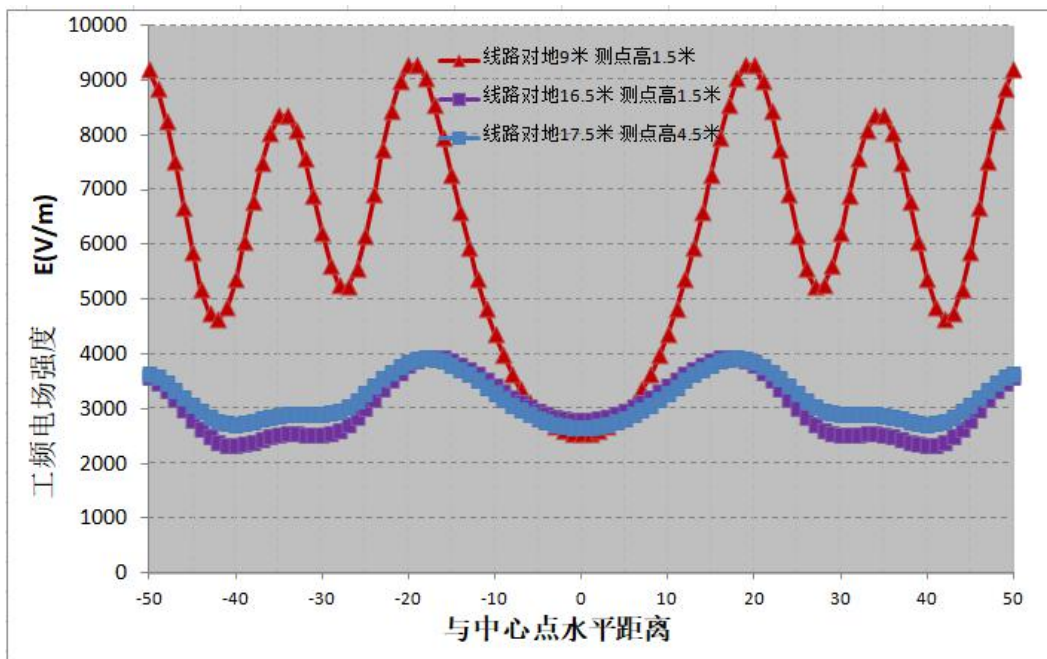
图 6-14 工频电场强度分布曲线图
