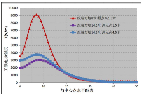
图 6.1-10 工频电场强度分布曲线图
