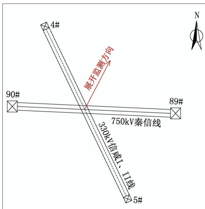
图 6.1-28 交叉跨越线路类比监测示意图
