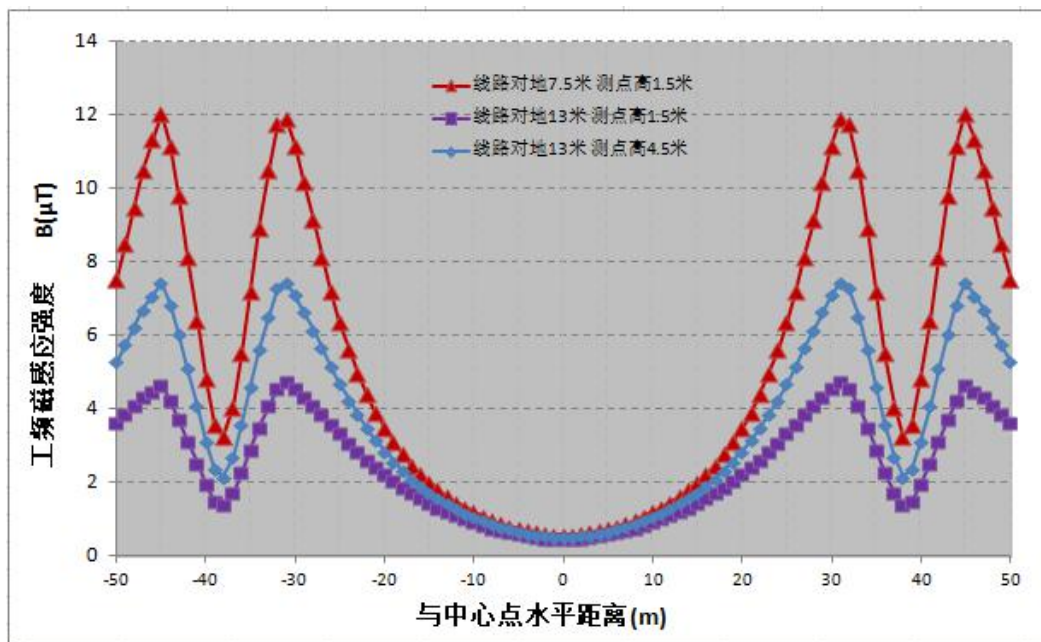
图 6.1-19 工频磁感应强度分布曲线图
