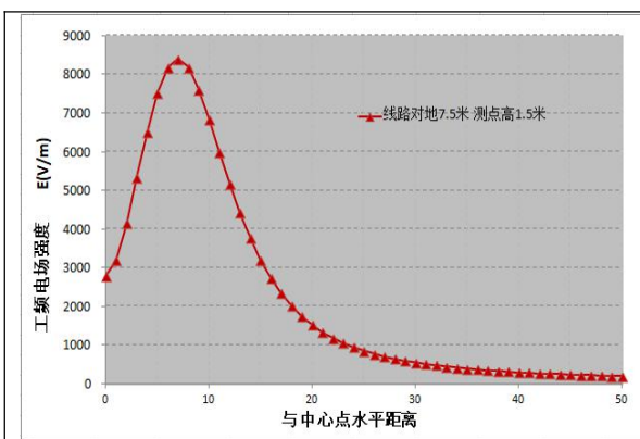
图 6.1-16 工频电场强度分布曲线图
