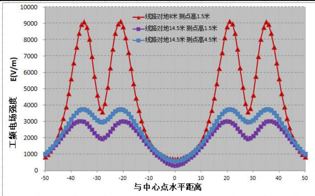
图 6.1-20 工频电场强度分布曲线图
