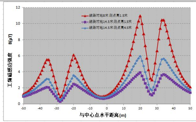
图 6.1-23 工频磁感应强度分布曲线图
