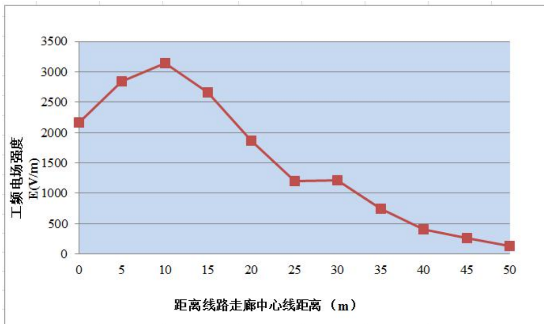
图 6.1-25 类比双回线路电场强度分布图
