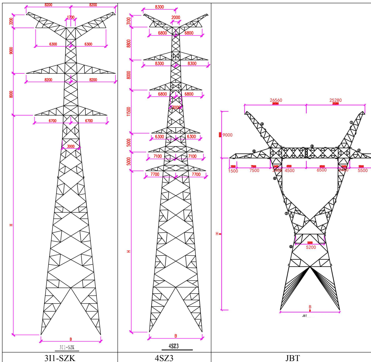
图 6.1-6 预测塔型图
