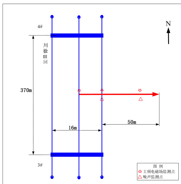
图 6.1-11 330kV 川徐Ⅲ回单回输电线路 3#~4#塔衰减监测断面示意图
