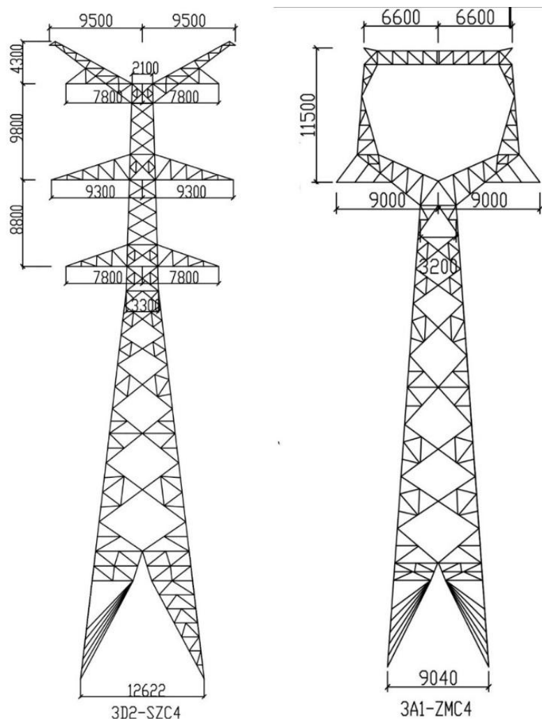
图 6.1-4 本工程预测塔型图
