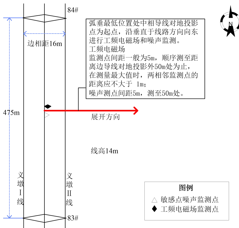
图 6.1-12 类比输电线路监测点位布设示意图
