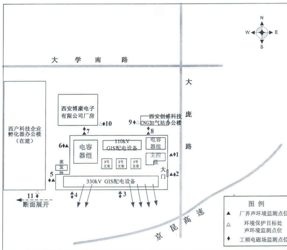
图 6.1-2 新盛 330kV 变电站监测点位示意图
