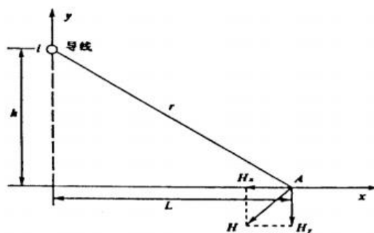
图 6.1-3 磁场向量图
