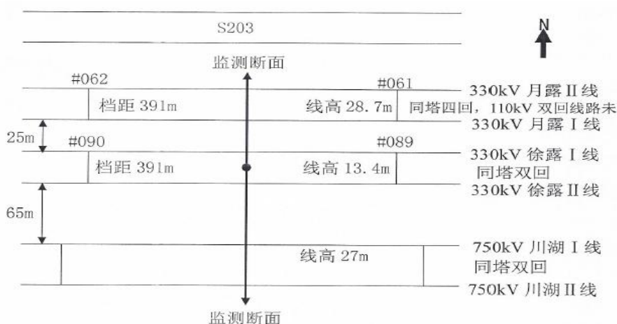
图 6.1-13 类比输电线路监测点位示意图
