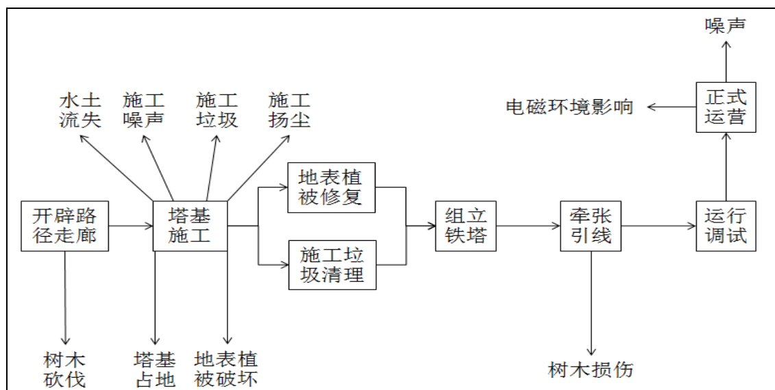
图 3-3 110kV 线路工艺流程及产污环节示意图
