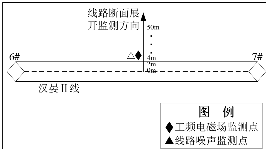
图7-2 输电线路断面展开监测点位布置示意图
