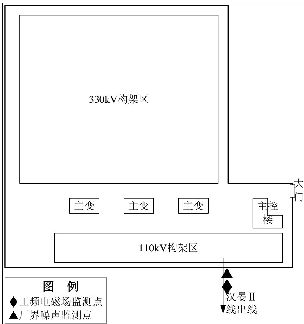
图7-1 汉中变汉晏II线出线间隔监测点位布置示意图
